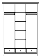
шкаф для платья и белья ГМ 8833, 2257 x 1555 x 642
