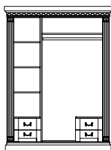
шкаф комбинированный ГМ 5823, 2110 x 1584 x 630
